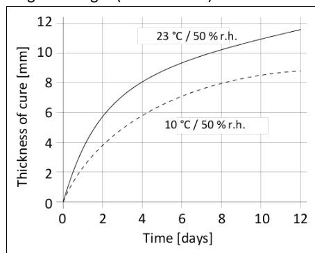
Schema 1: Uithardingssnelheid Sikaflex®-290 DC PRO
