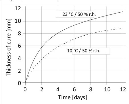
Schema 1: Doorhardingsnelheid van Sikaflex®-221
